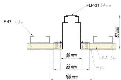
چراغ آویز
